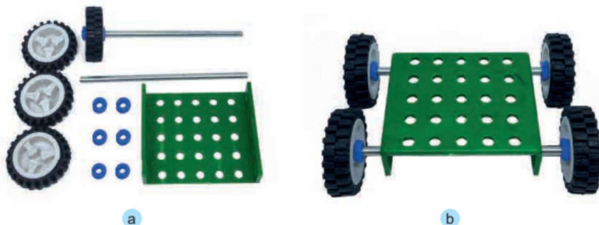
Hình 4 Chân robot và các chi tiết
