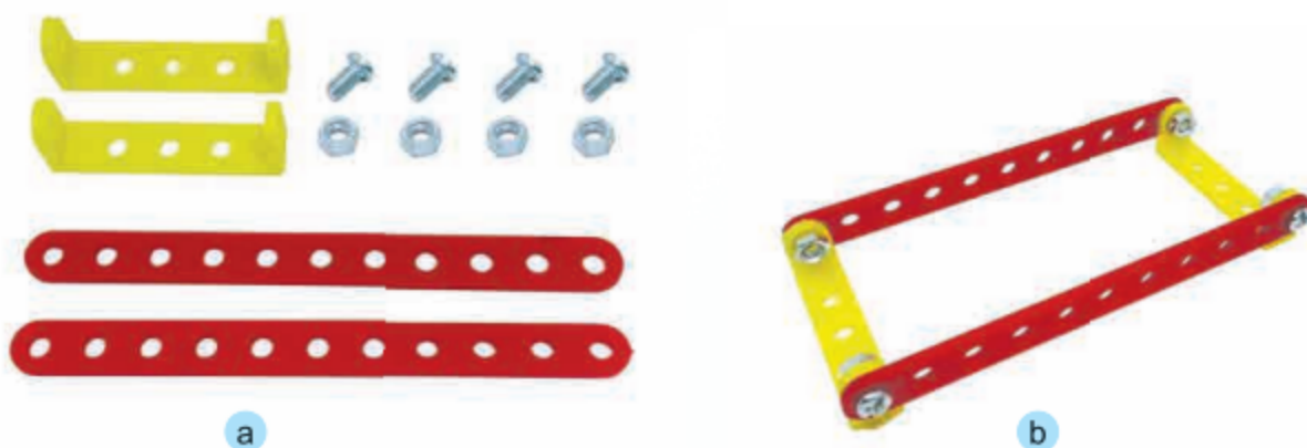
Hình 3 Ghế ngồi bập bênh và các chi tiết
