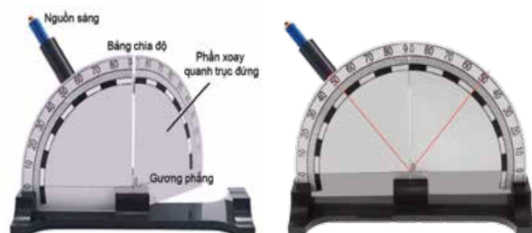
▲ Hình 16.3. a) Bố trí thí nghiệm; b) Quan sát tia sáng tới và tia sáng phản xạ khi nửa bên phải của bảng chia độ cùng mặt phẳng với nửa bên trái
